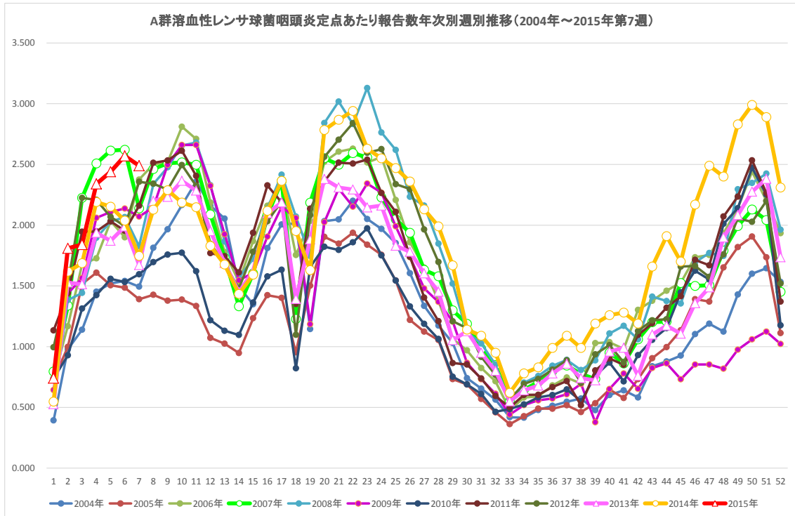
図. A群溶血性レンサ球菌咽頭炎小児科定点あたり報告数年次別週別推移（2004年～2015年第7週）
